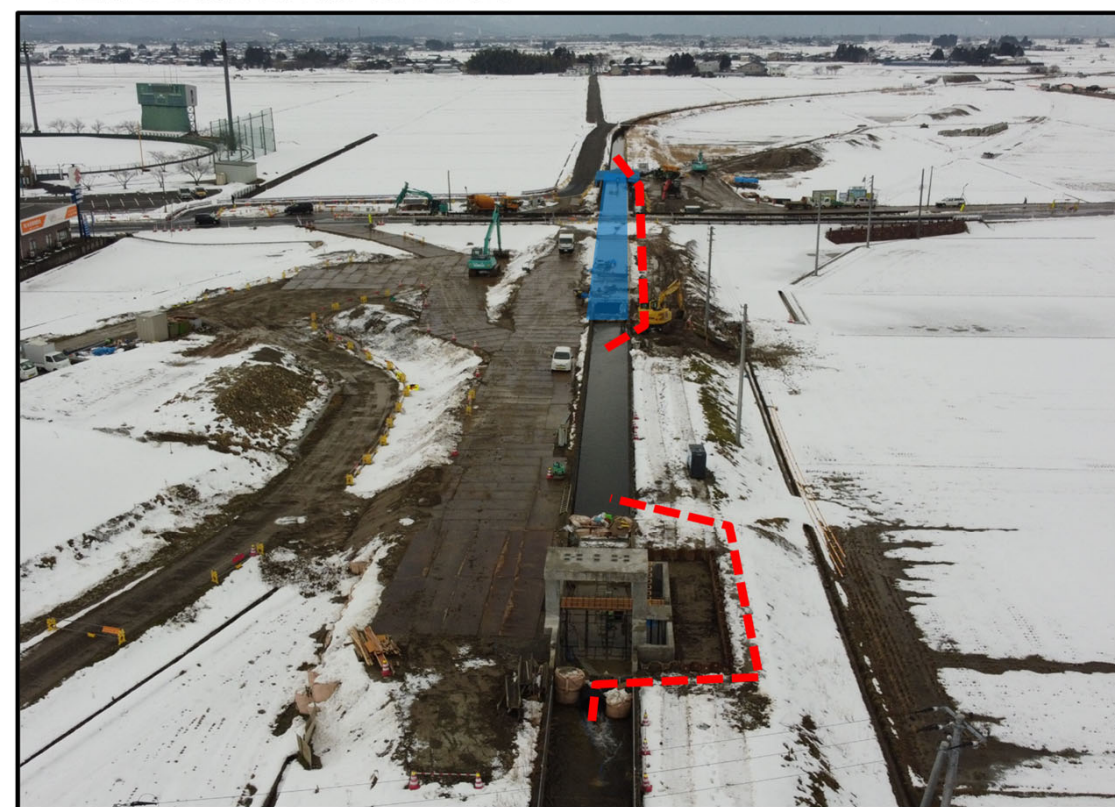
仮水路φ900 赤破線 L=160m カルバート 青着色 L=102m
