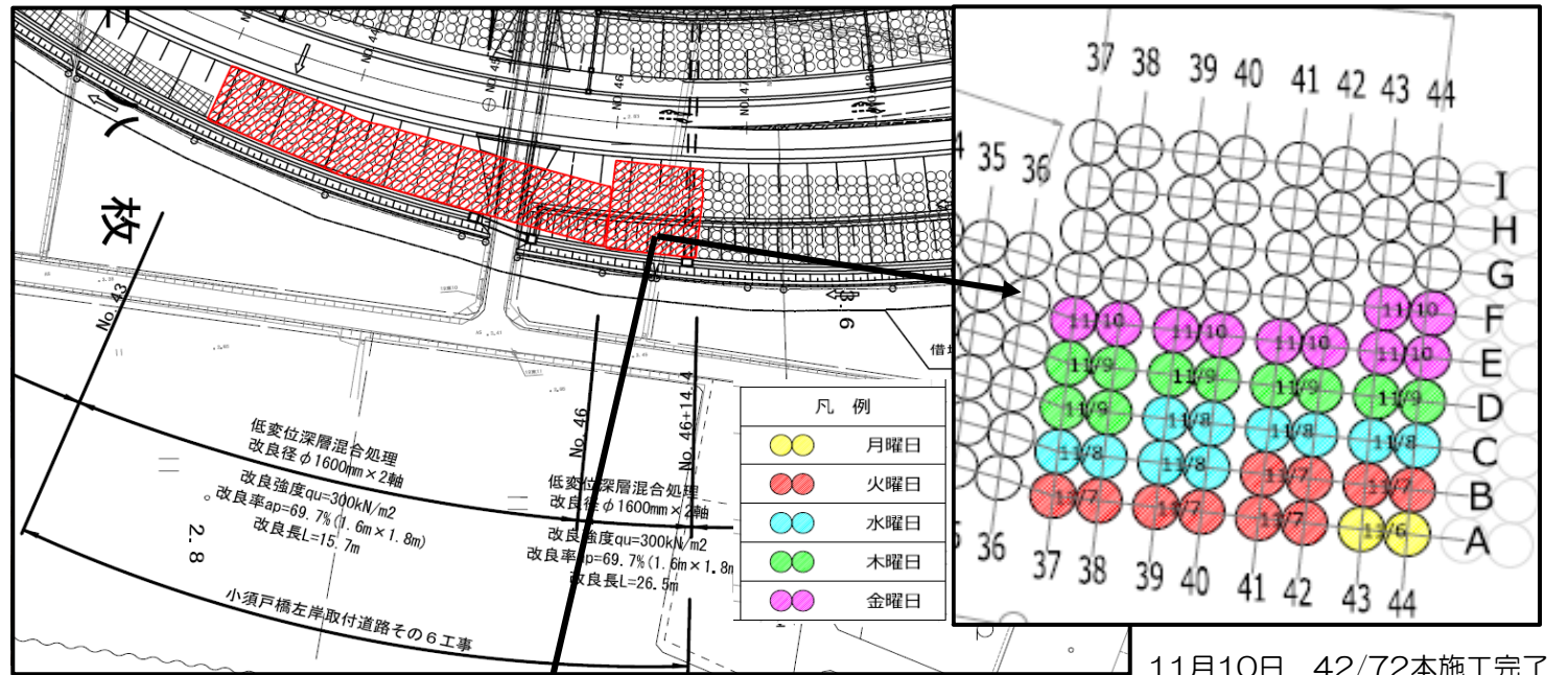
地盤改良工
